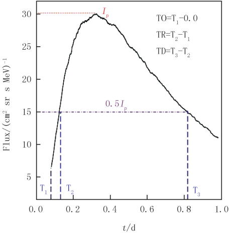
图 1 太阳高能粒子通量随时间变化图 Fig.1 Solar energetic particle flux with time
