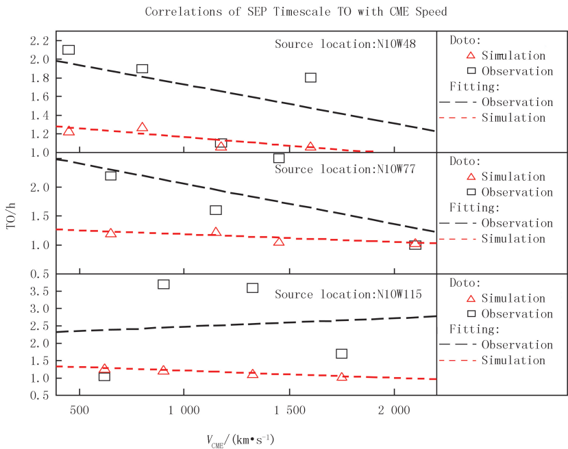
图 4 数值模拟方法下 SEP 时间尺度 TO 与 CME 速度关系数值模拟与观测对比图
