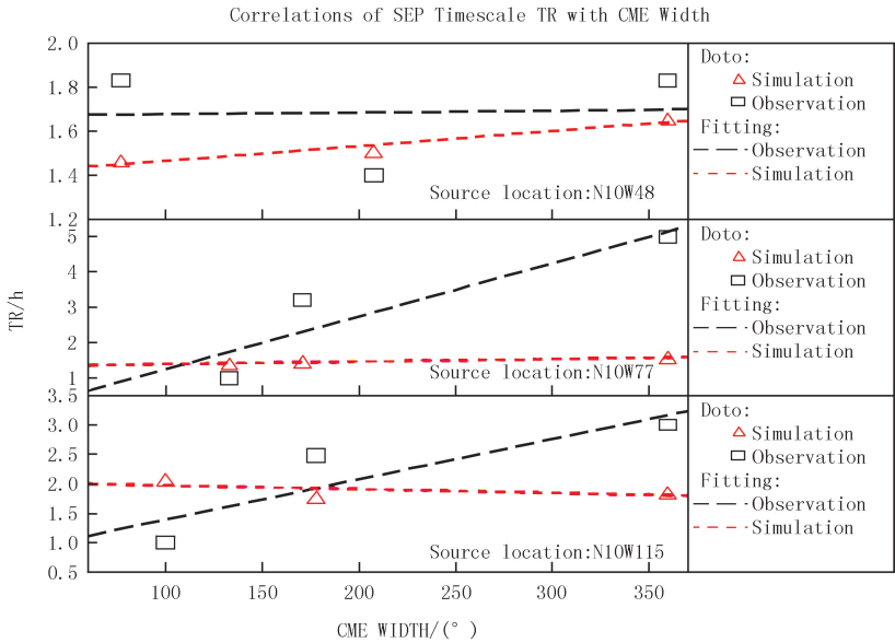
图 3 数值模拟方法下 SEP 时间尺度 TR 与 CME 宽度关系数值模拟与观测对比图
