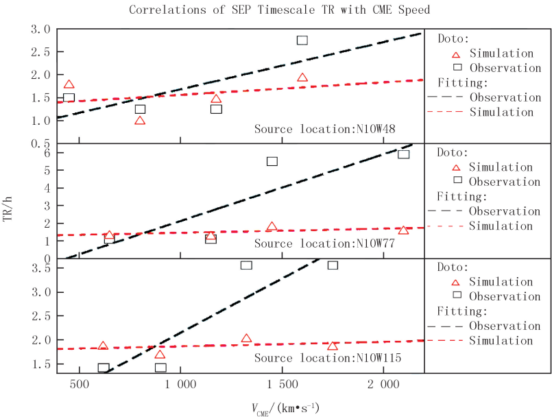
图 2 数值模拟方法下 SEP 时间尺度 TR 与 CME 速度关系数值模拟与观测对比图 Fig.2 Comparison of SEP timescale TR and CME velocities with simulation and observation under numerical simulation method
