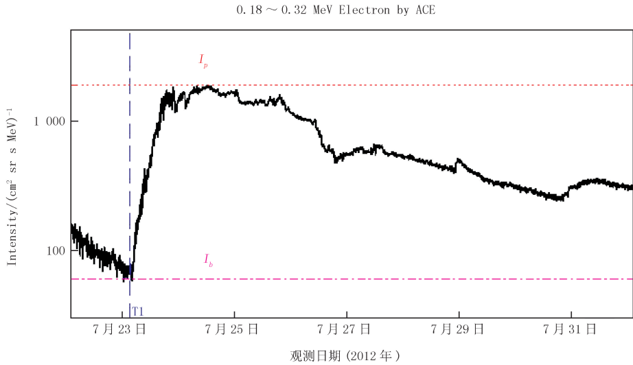
图 6 由 ACE 卫星观测的能量在 0.18 ~ 0.32 MeV 电子的强度随时间变化图 Fig.6 The intensity of energetic electrons observed by ACE satellite in 0.18-0.32 MeV varies with time
