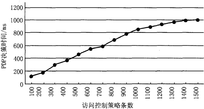
图5 访问控制策略数量与PDP决策时间的关系
