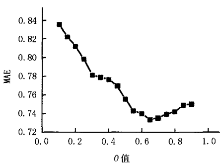
图 2 意见质量 O 对 MAE 的影响
