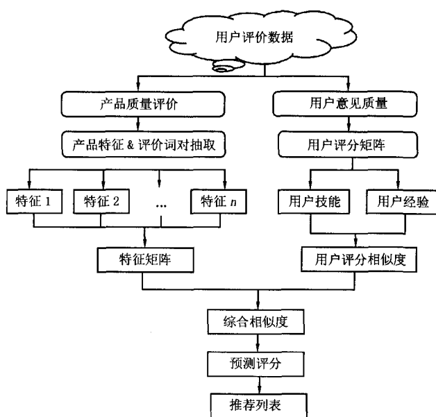
图1 推荐算法整体框架
