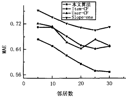
图 3 邻居数对 MAE 值的影响
