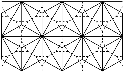
图 1 实线构成的晶格为 centered-triangular 晶格, 虚线构成的晶格为 3-12 晶格
