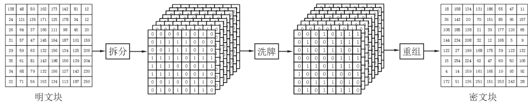
图2 块以二进制进行位平面拆分加密的流程图
