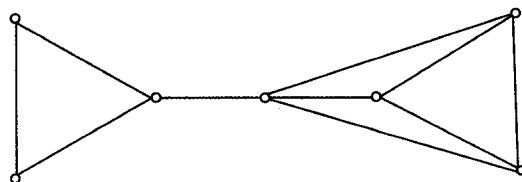
图4 与图 H 同构的图
