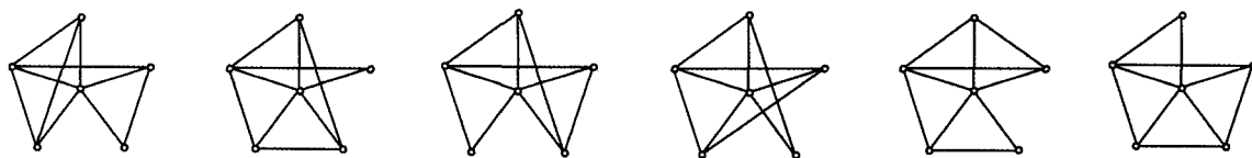
图3 与 H 同构的图
