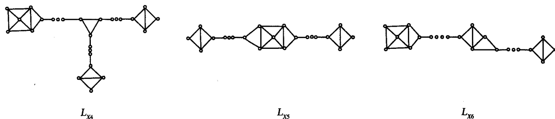
图8 X_4, X_5, X_6 的线图
