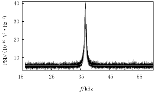
黑线:自旋噪声谱实验数据;灰线:洛伦兹拟合噪声谱曲线. 图3 快速傅里叶变换后的自旋噪声谱 Fig.3 Spin noise spectrum from FFT analysis
