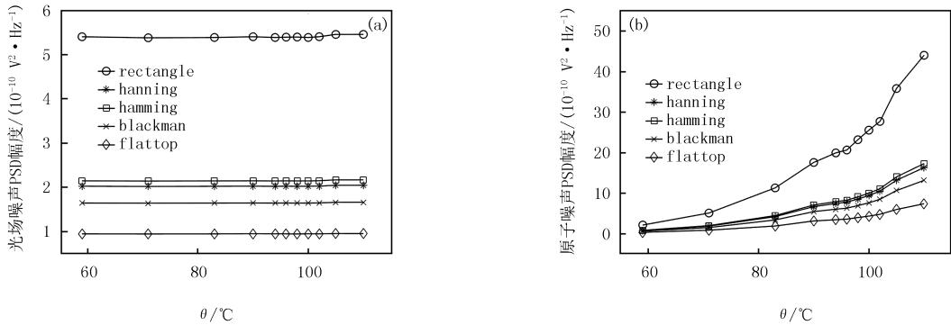
图4 光场噪声(a)和原子自旋噪声(b)在不同窗函数下随温度变化图 Fig.4 Optical noise(a) and spin noise(b) versus temperature under different window functions
