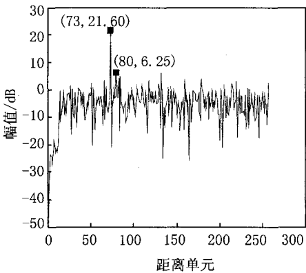
图 6 均衡长度为19时的输出信号
