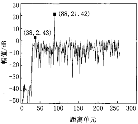
图 7 均衡长度为49时的输出信号
