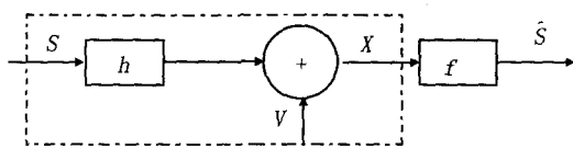
图 3 信道均衡中的信号模型
