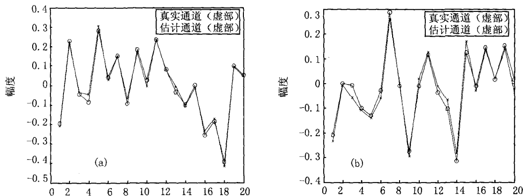
图 4 多径信道估计与真实信道对比
