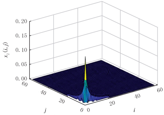
图4 系统(1)状态变量 x_2(i, j) 轨迹 Fig.4 State x_2(i, j) trajectory of the system(1)
