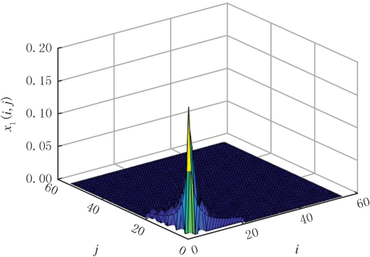
图1 系统(1)状态变量 x_1(i, j) 轨迹 Fig.1 State x_1(i, j) trajectory of the system(1)
