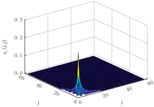
图3 系统(1)状态变量 x_1(i, j) 轨迹 Fig.3 State x_1(i, j) trajectory of the system(1)
