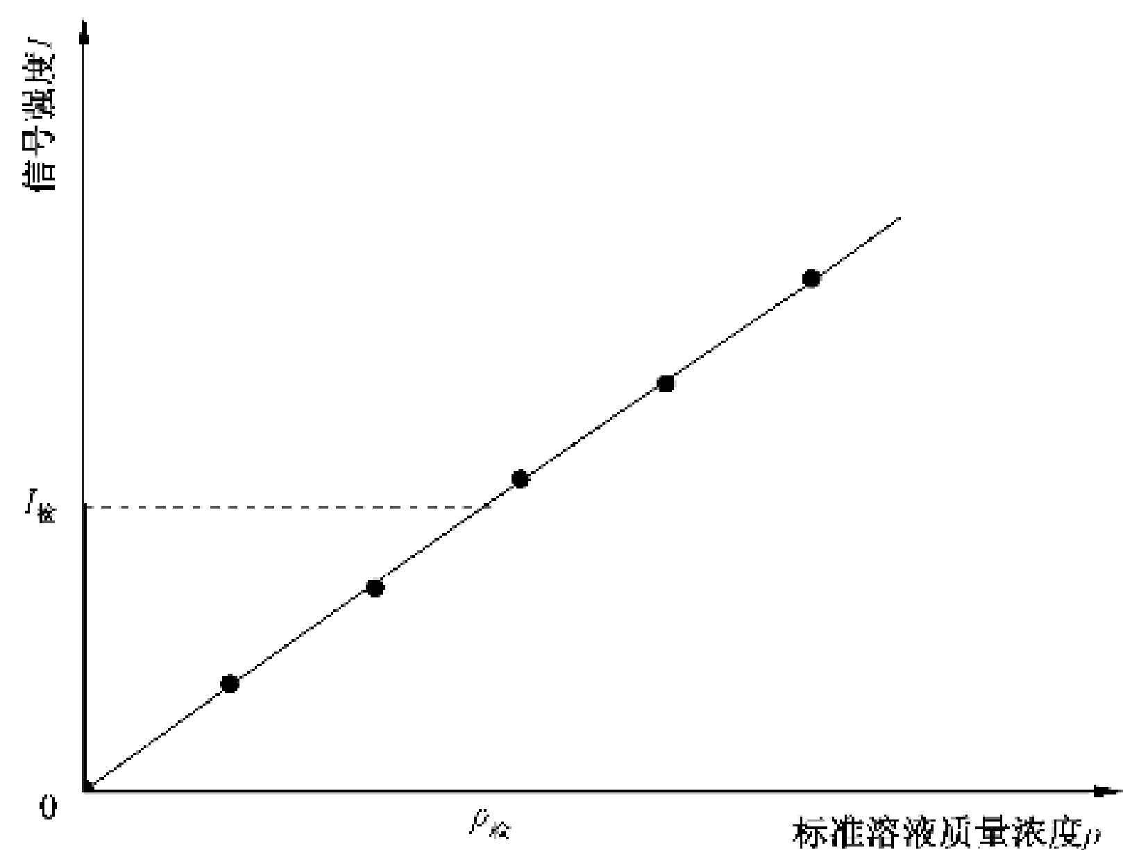
图 1 标准曲线法的校准曲线
