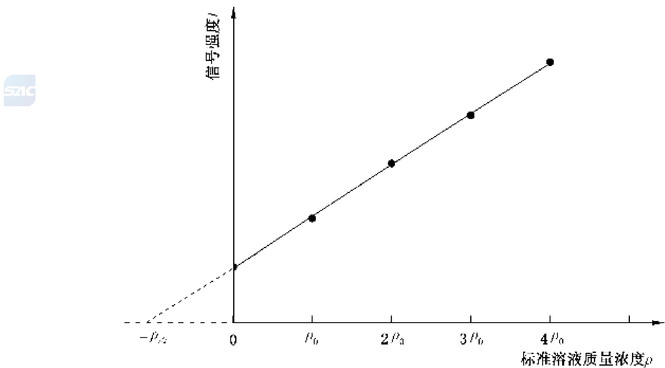
图 2 标准加入法的校准曲线
