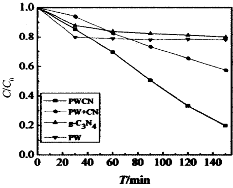
图5 模拟太阳光下催化剂的光降解曲线
