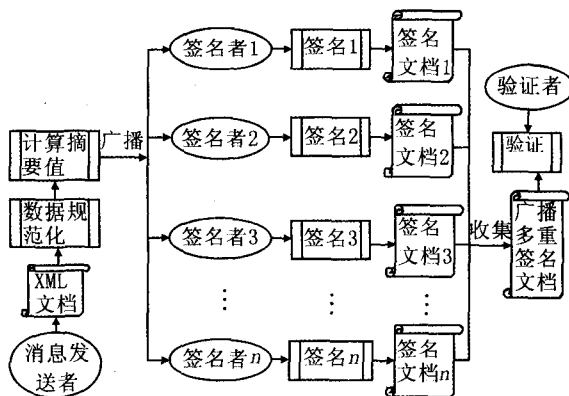
图2 XML广播多重签名模型
