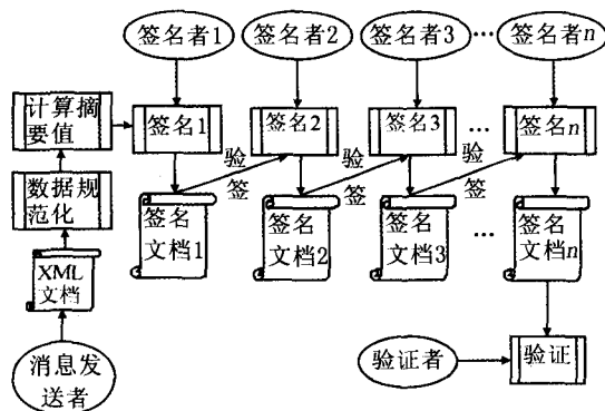
图1 XML有序多重签名模型
