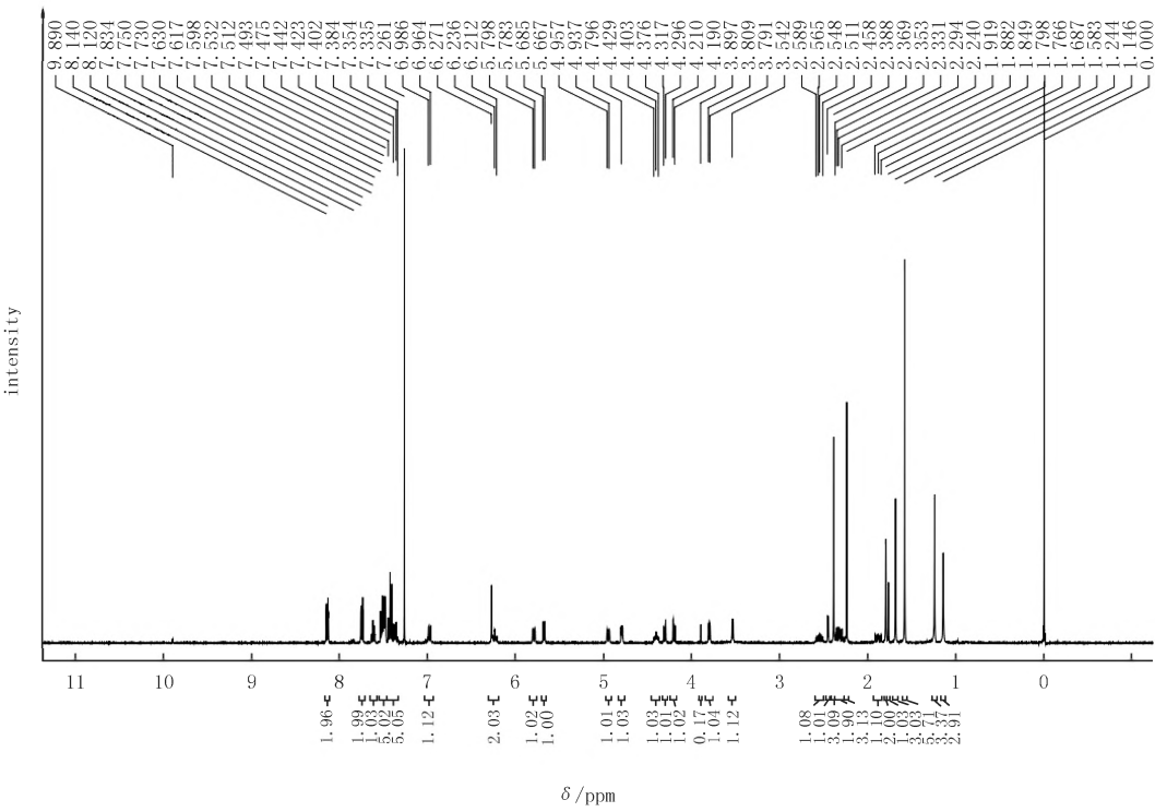
图4 合成制备紫杉醇的 ^1\text{H} -NMR图谱 Fig.4 ^1\text{H} -NMR of synthesized taxol
