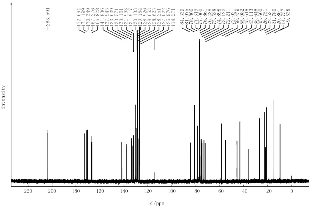
图5 合成制备紫杉醇的 ^{13}\text{C} -NMR图谱 Fig.5 ^{13}\text{C} -NMR of synthesized taxol
