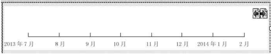
图 4 时间轴控件
