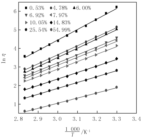
图 3 不同含水量条件下, HEtHex(TFS) 的 \ln \eta 值随 1000/T 的变化关系图 Fig.3 Plot of \ln \eta vs. 1000/T for HEtHex (TFS) at different water contents
