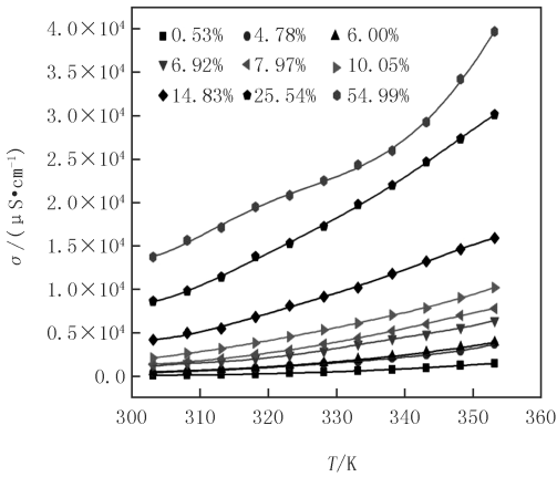
图 4 不同含水量条件下, HEtHex(TFS) 的电导率 \sigma 与温度 T 的变化关系 Fig.4 Plot of \sigma vs. T for HEtHex(TFS) at different water contents
