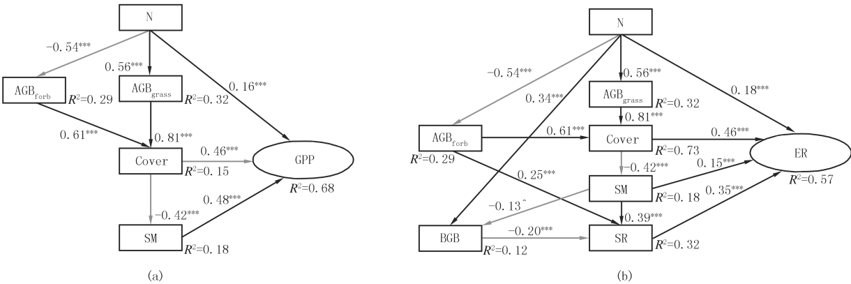
(a) 氮素添加通过植物地上生物量、盖度、土壤湿度直接和间接对温带典型草原生态系统总初级生产力(GPP)产生影响的结构方程模型; (b) 氮素添加通过植物地上生物量、盖度、土壤湿度直接和间接对生态系统呼吸(ER)产生影响的结构方程模型. 黑色实线代表正相关, 灰色实线代表负相关. 模型拟合结果:对于GPP, \chi^2=10.658 , df=7 , P=0.15 ;对于ER, \chi^2=24.568 , df=14 , P=0.08 .
